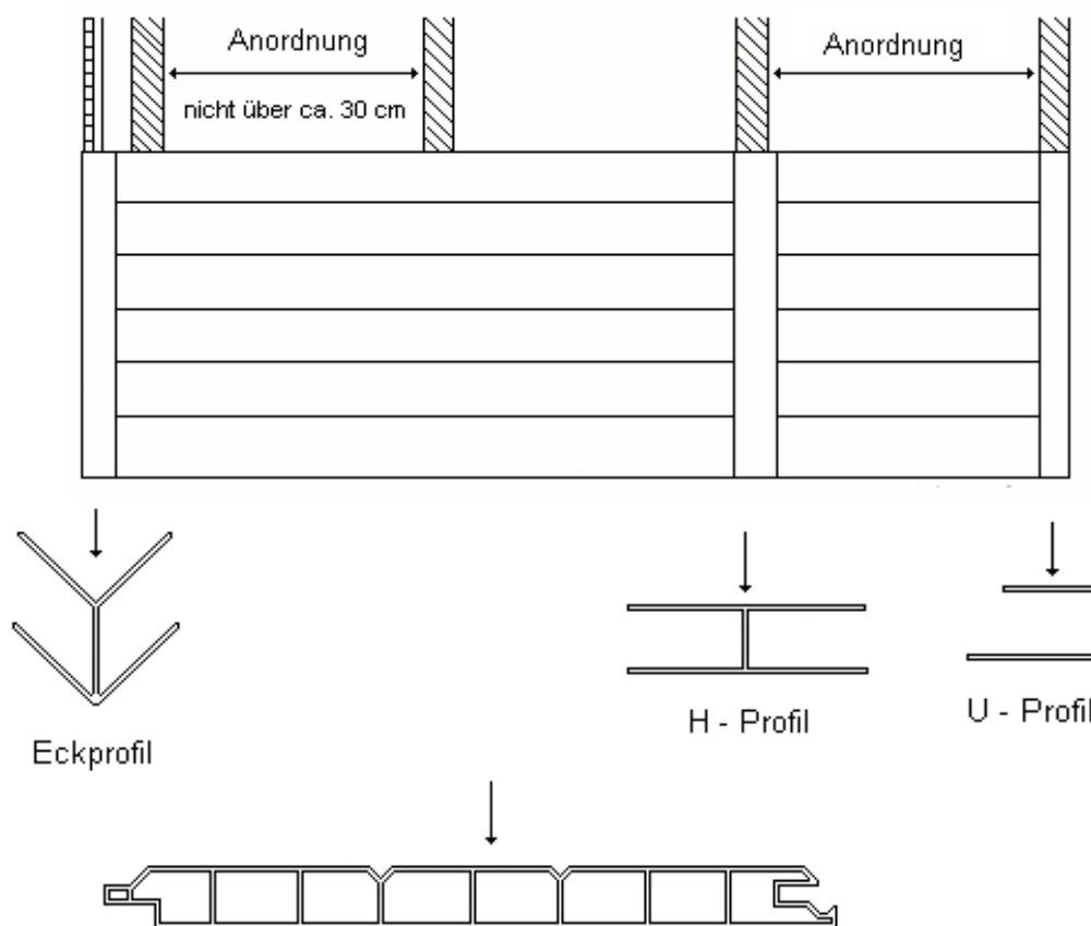
Verkleidungsprofil - VP 200
